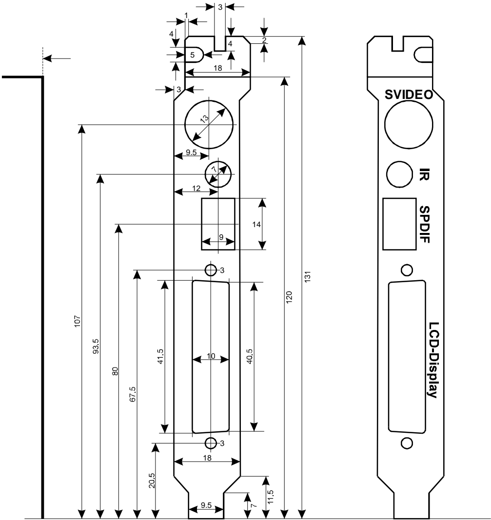
Blechabwicklung
